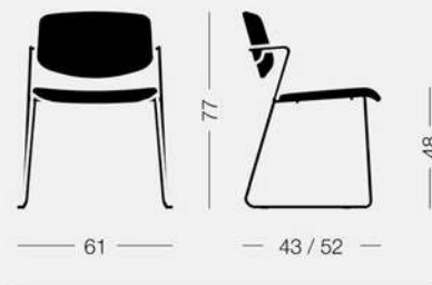
Serpentine 1C00 6,8 kg 0,36 m³ 2 pz Poltroncina, struttura in acciaio Armchair, steel structure
