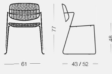
Serpentine Outdoor 1C01 6,00 kg 2 pz Poltroncina, struttura in acciaio Armchair, steel structure
